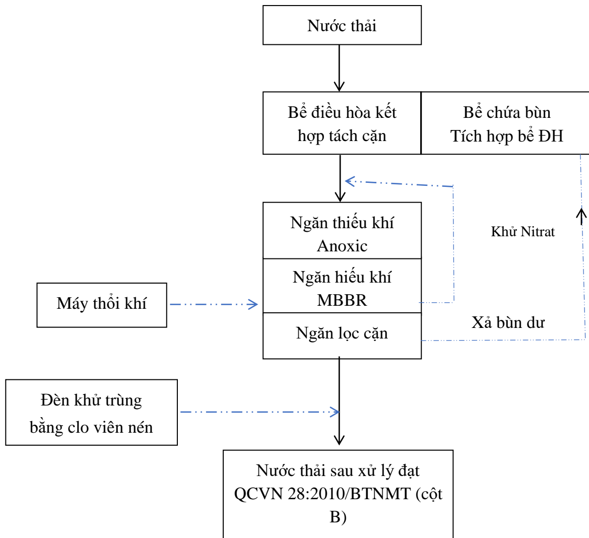
Hình 3.5. Sơ đồ công nghệ hệ thống XLNT trạm y tế xã Mường Cang
