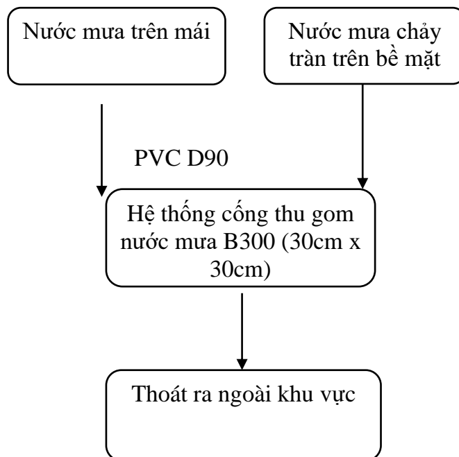
Hình 3.1. Sơ đồ thu gom nước mưa của trạm y tế xã Mường Cang
