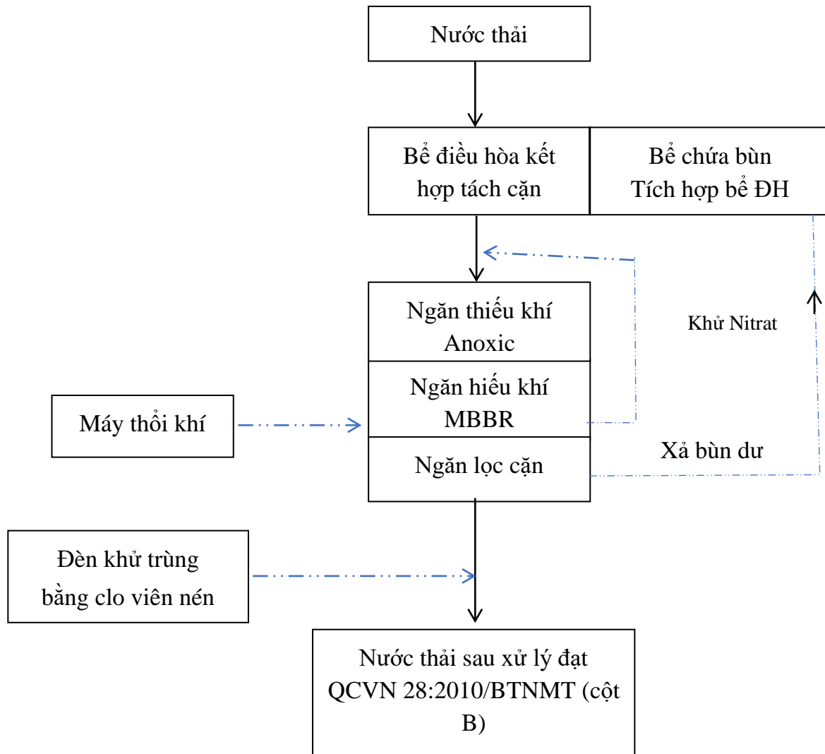
Hình 3.5. Sơ đồ công nghệ hệ thống XLNT trạm y tế thị trấn Than Uyên
