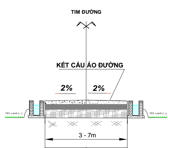
MẶT CẮT 3-3
