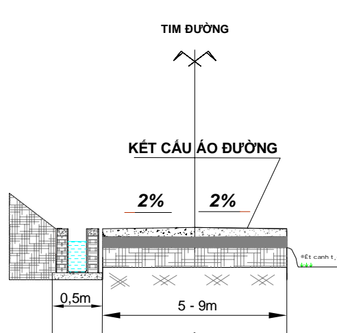
MẶT CẮT 2-2
