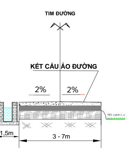
MẶT CẮT 5-5
