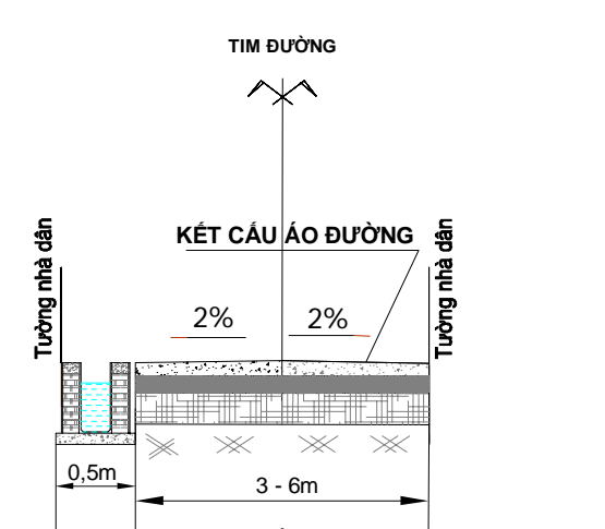
MẶT CẮT 4-4
