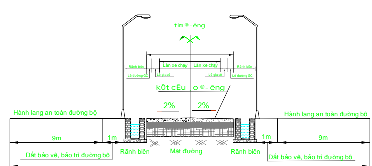
MẶT CẮT 1-1 (ĐƯỜNG QUỐC LỘ NGOÀI ĐỒ THỊ)
