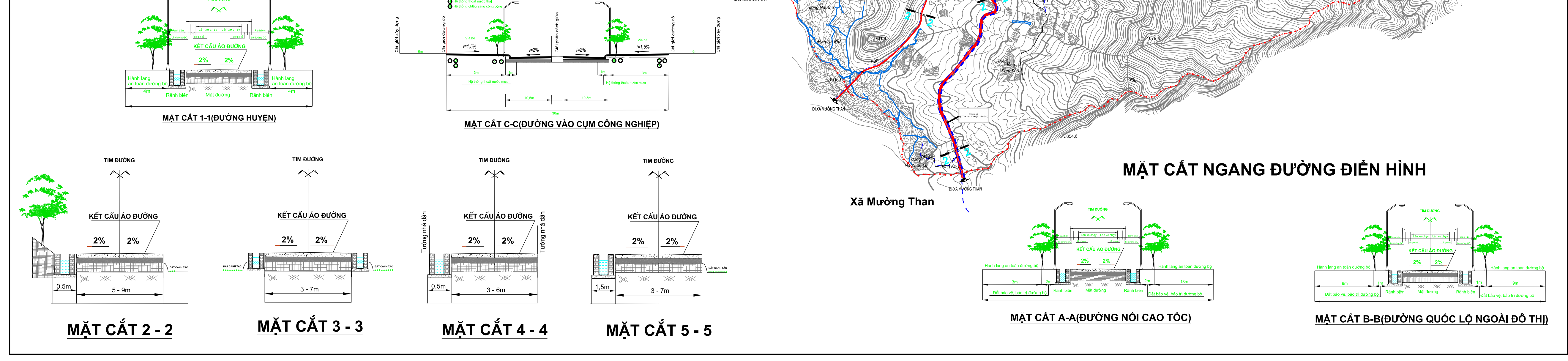
MẶT CẮT NGANG ĐƯỜNG ĐIỆN HÌNH
